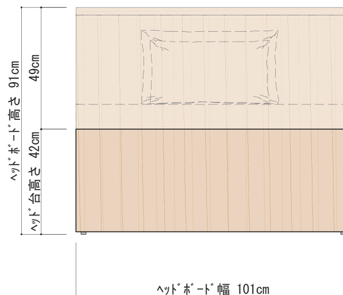
正面
