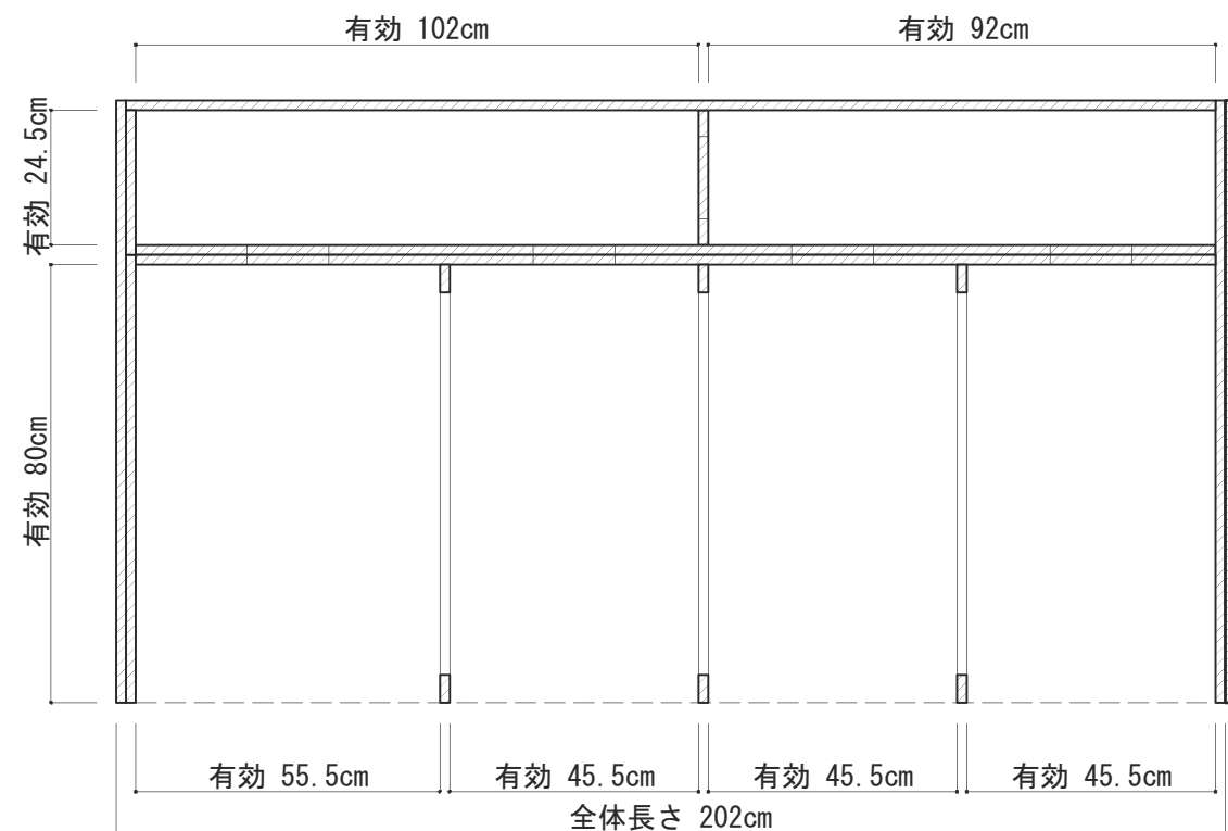
平断面
