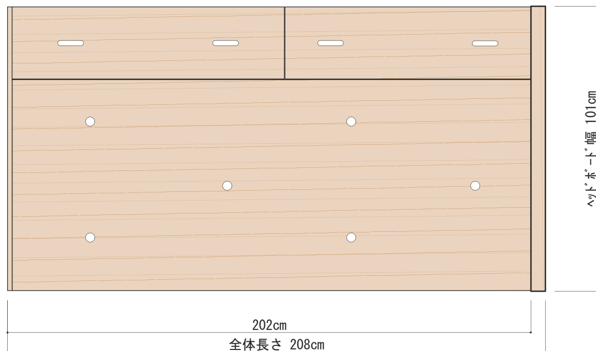
平面
