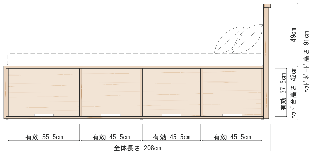
側面
